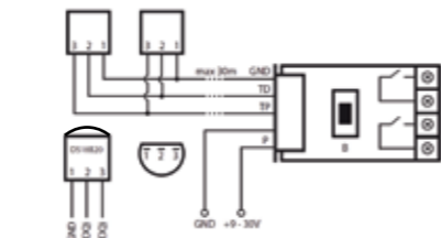
Collegamento a sensori di temperatura DS18B20
