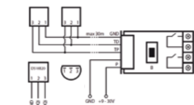
Verbinding met DS18B20 temperatuur sensoren
