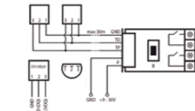
Anschluss an DS18B20 Temperatursensor
