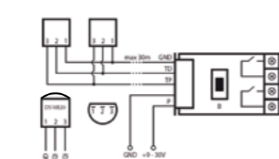
Connexion aux capteurs de température DS18B20
