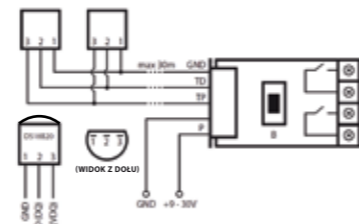
Połączenie czujników temperatury DS18B20
