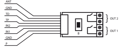
Voorbeeld van een verbinding met een bekabelde sensor
