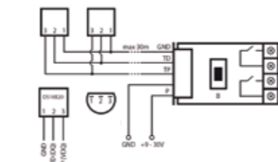
Připojení k teplotním čidlům DS18B20
