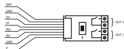
Przykładowe połączenie z czujnikiem przewodowym
