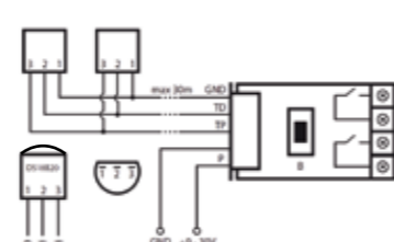
Exemplo da ligação a um sensor cabeado
