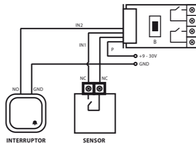
Exemplo da ligação a um sensor cabeado
