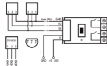
Conexión de sensores de temperatura DS18B20
