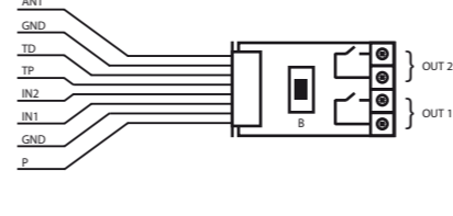
Пример подключения к проводному датчику
