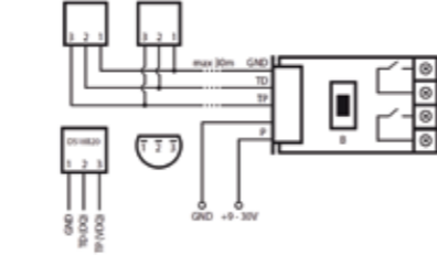
Подключение к температурным датчикам DS18B20
