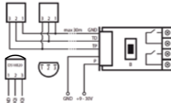
Anslutning till DS18B20 temperaturgivare
